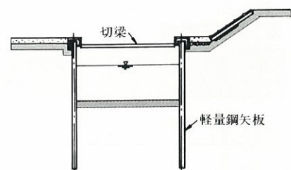
切梁式護岸
