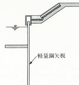
自立式護岸
