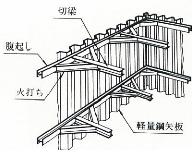
土留め
