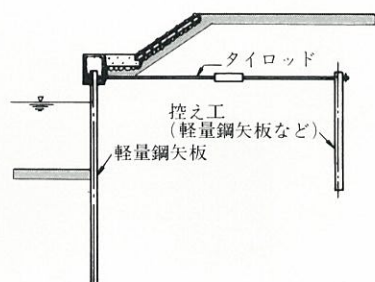
タイロッド式護岸
