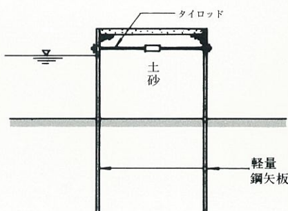
仮締切
